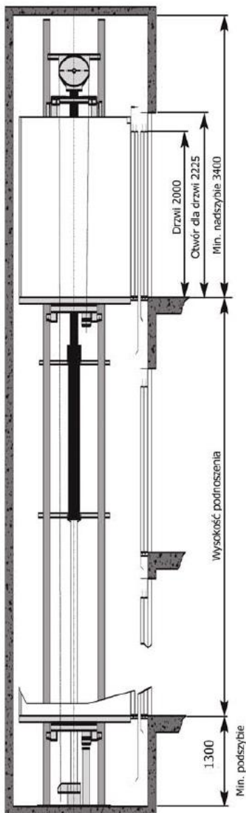
PRZEKRÓJ PIONOWY
