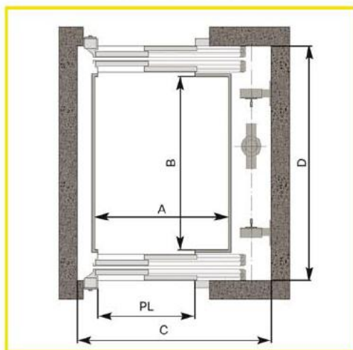
PRZEKRÓJ POZIOMY 2 WEJŚCIA (PRZELOT)
